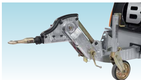
Параллельно установленное дышло с тормозом наката и буксировочной петлёй
